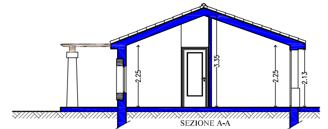
SEZIONE A-A
