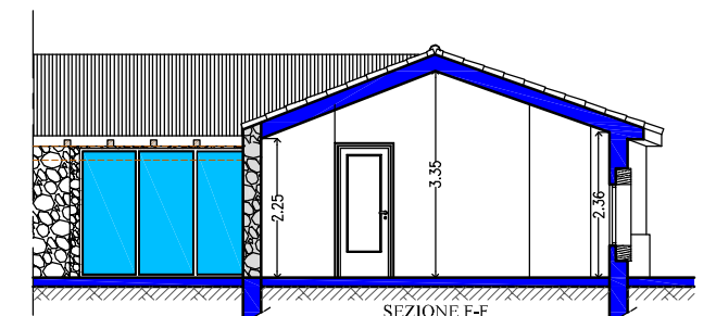
SEZIONE F-F
