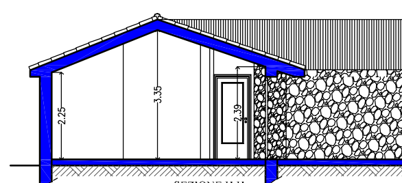
SEZIONE H-H
