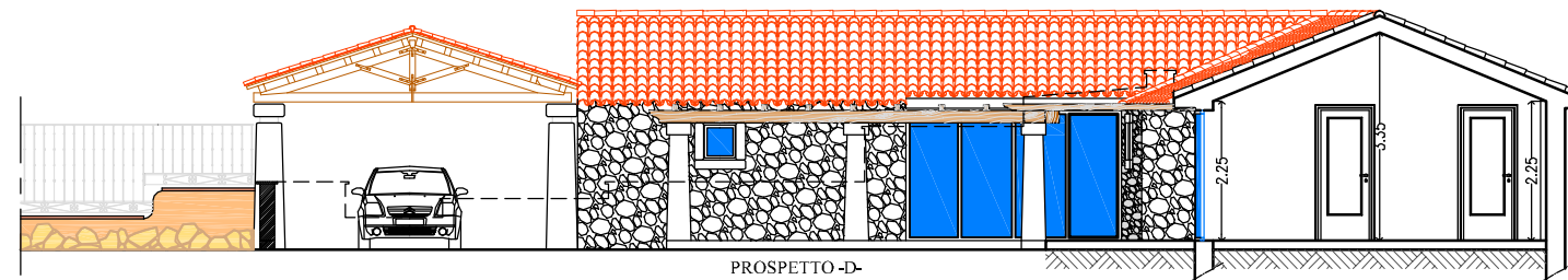
PROSPETTO-D-
