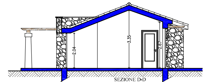
SEZIONE D-D
