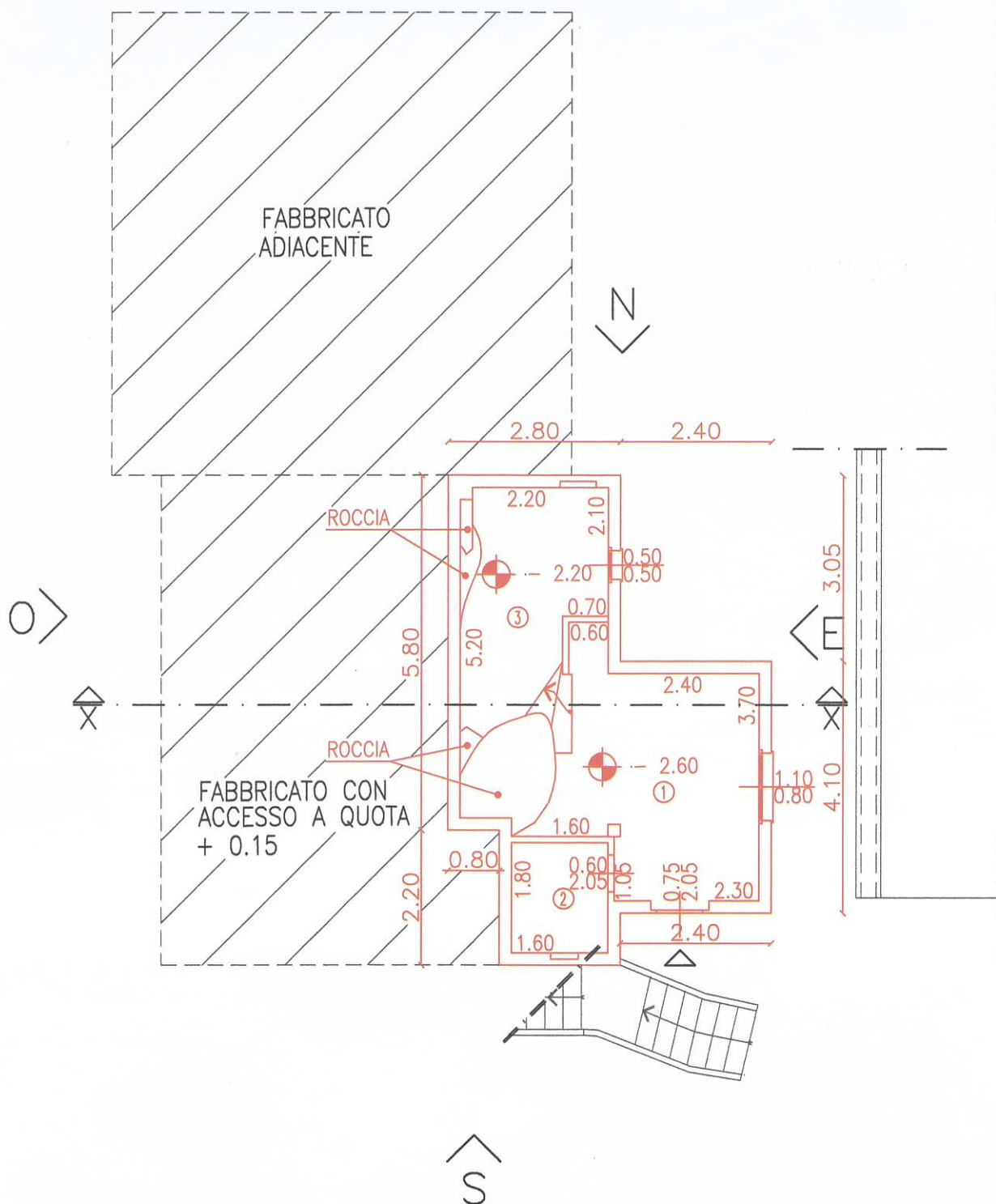
PIANTA QUOTATA (Dopo L' Abuso) Rapp. 1 : 100
